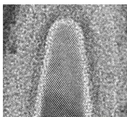
Затвор транзистора 22 нм (точки - атомы кремния)
